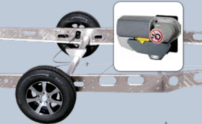
Drehstabfederachse mit Längslenkertechnik inkl. Montagevorbereitung für TRUMA-Mover
